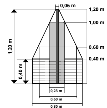
Fig 5 : Abaque de détection des obstacles
